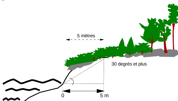
Figure 2.7e : Talus
